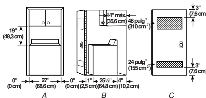
A. Vista frontal B. Vista lateral C. Puerta del armario con celosías de ventilación
